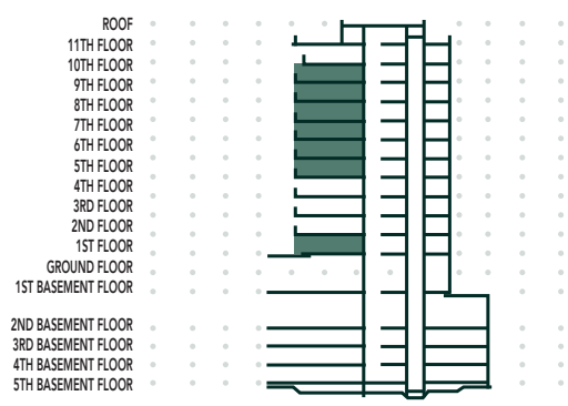
A-D, A-F BLOCKS SECTION
